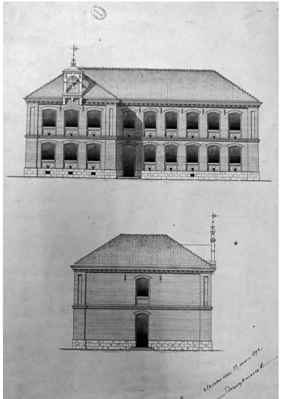
Projekt budynku prywatnego z 1892 r. autorstwa S. Zaremby
